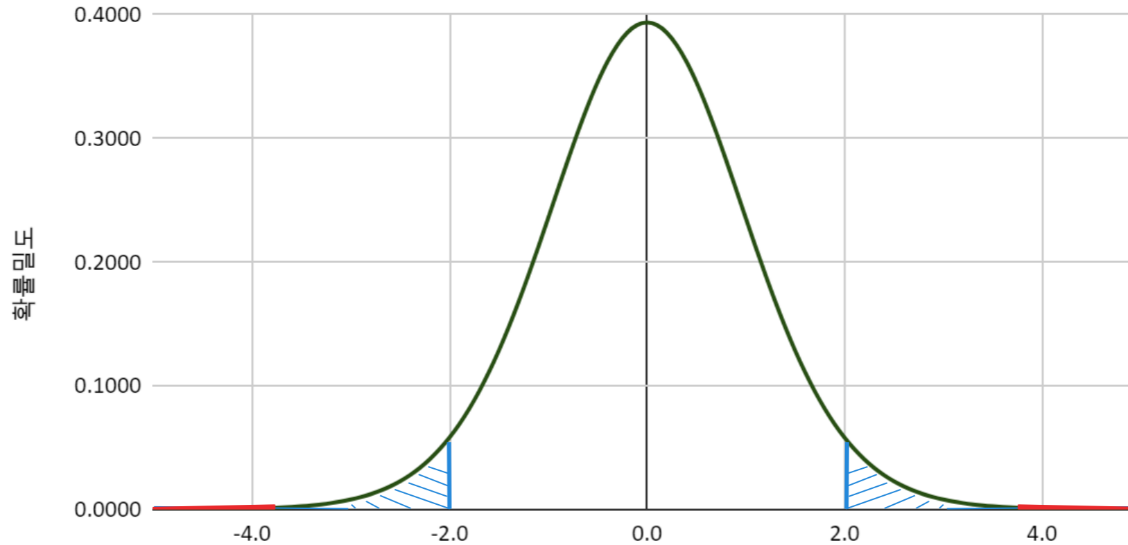
t분포(자유도 19)
